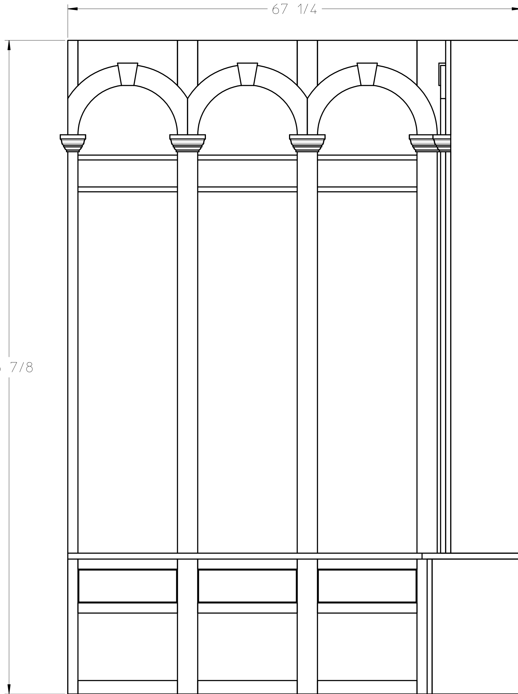
FRONT1 SCALE 1:8
