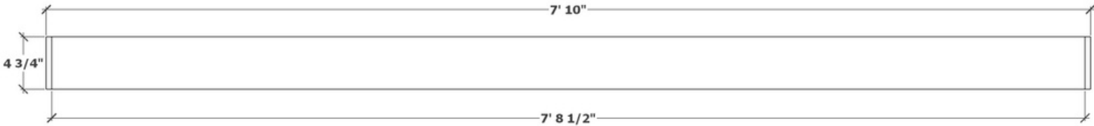
BOTTOM PANEL - QTY 1
