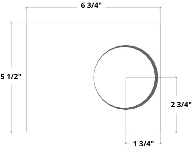
BOX BOTTOM - QTY 1
