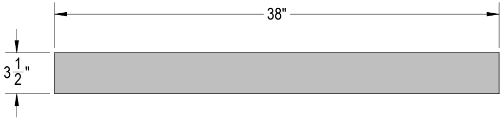
②② BED SLATS MATERIAL: 1 X 4 PINE QTY: 11
