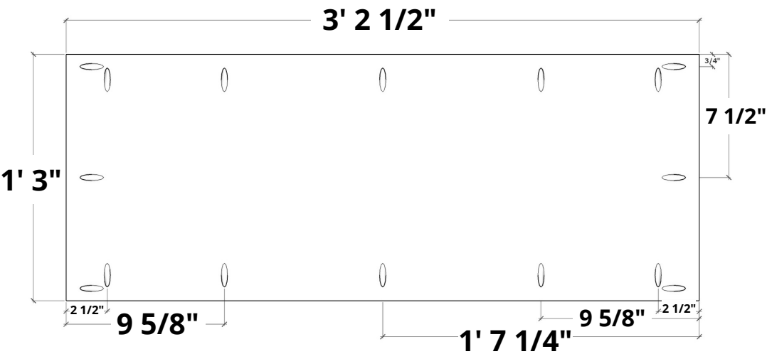
BOTTOM PANEL - QTY 1
