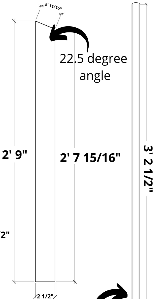
FRAME SIDES - QTY 4
